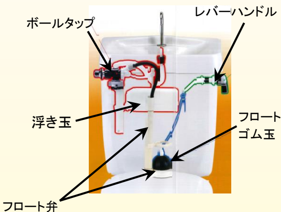
タンクの構造と部品名称
